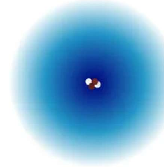
ERWIN SCHRÖDINGER, 1926
